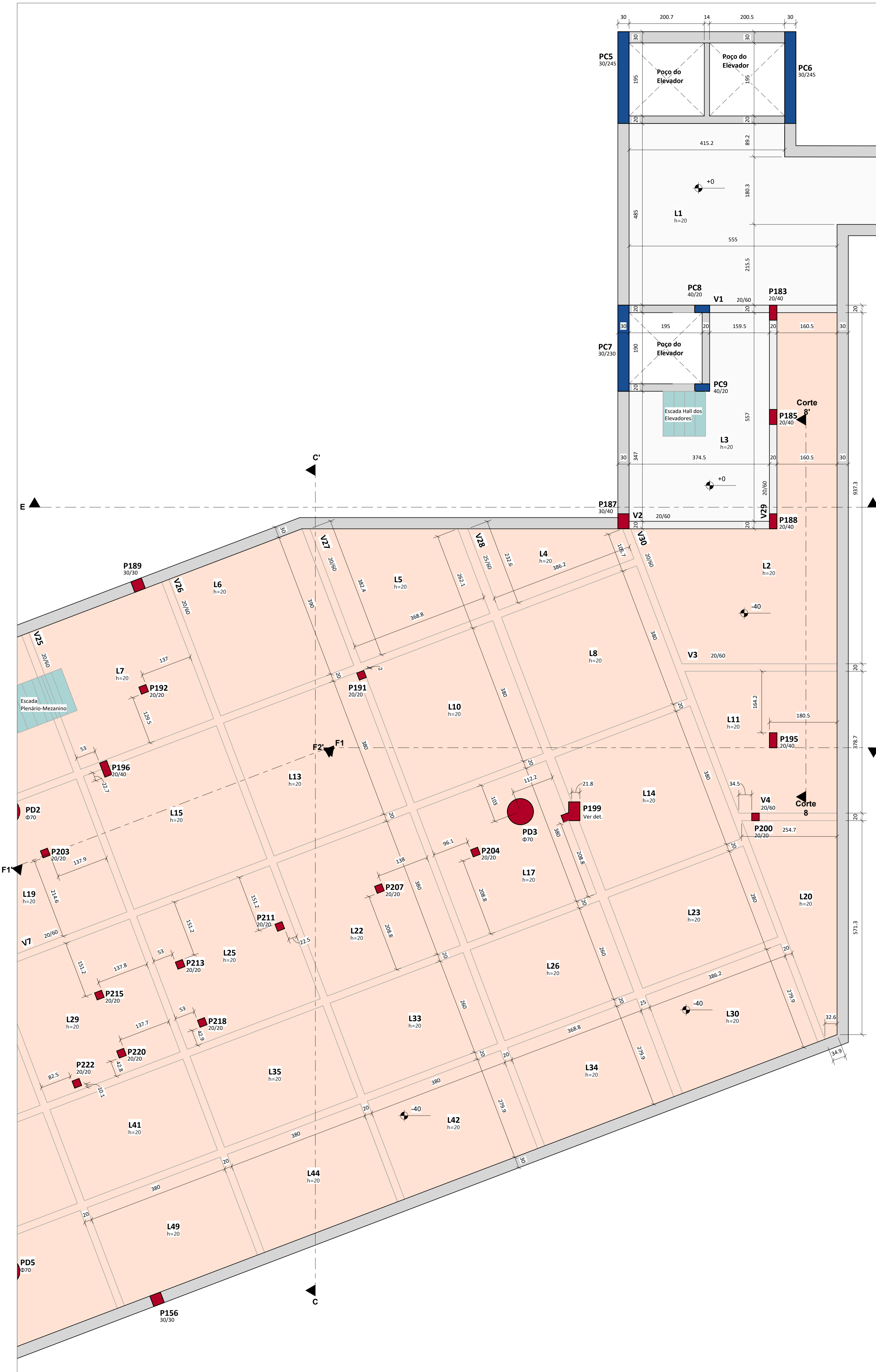
Forma do Pavimento: 00-Subsolo - I-2 Escala: 1 : 50
